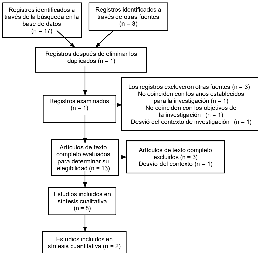
Figura 1 Diagrama del método PRISMA
